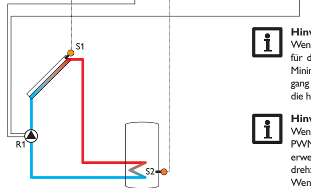
Beispiel für den elektrischen Anschluss einer Hocheffizienzpumpe
