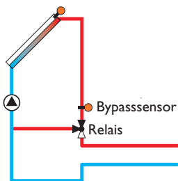
Variante Ventil:
