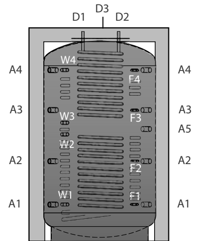
Hygienespeicher mit zwei Wärmetauschern
