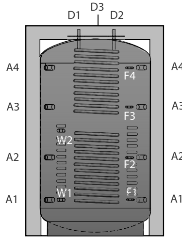
Hygienespeicher mit einem Wärmetauscher
