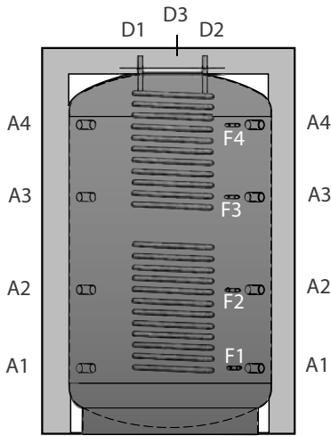
Hygienespeicher ohne Wärmetauscher
