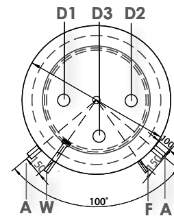
Draufsicht Hygienespeicher Typ KE, KER, KER2 100° Anschlüsse
